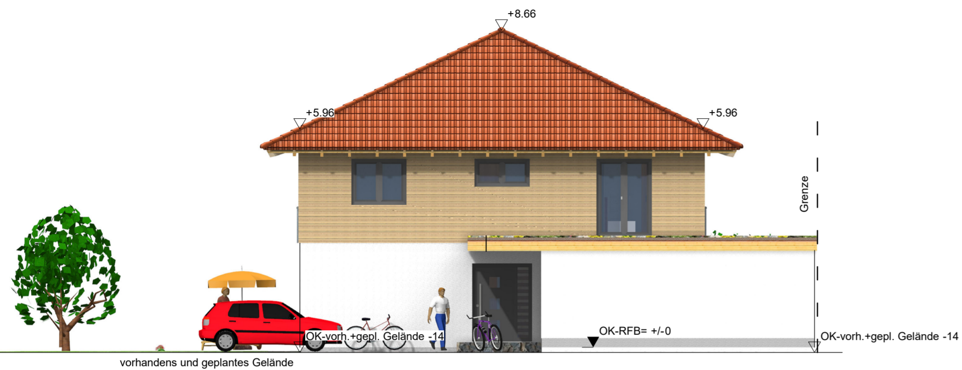
ANSICHT - Osten
