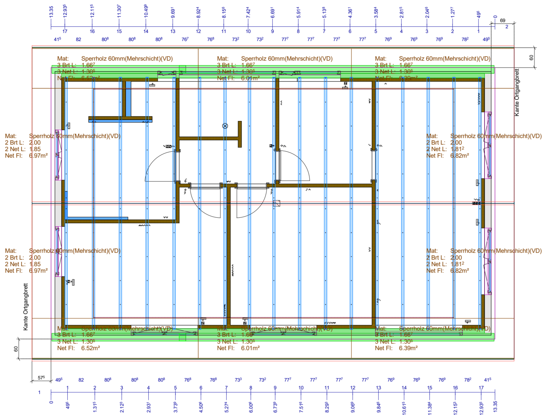
Aufdachsparrenlage
