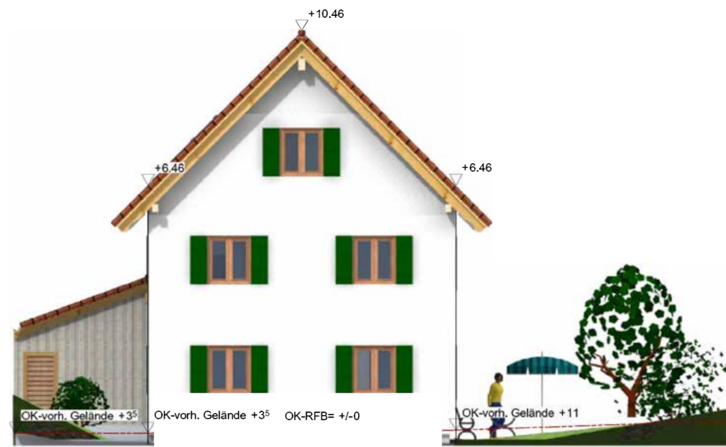
ANSICHT - Westen
