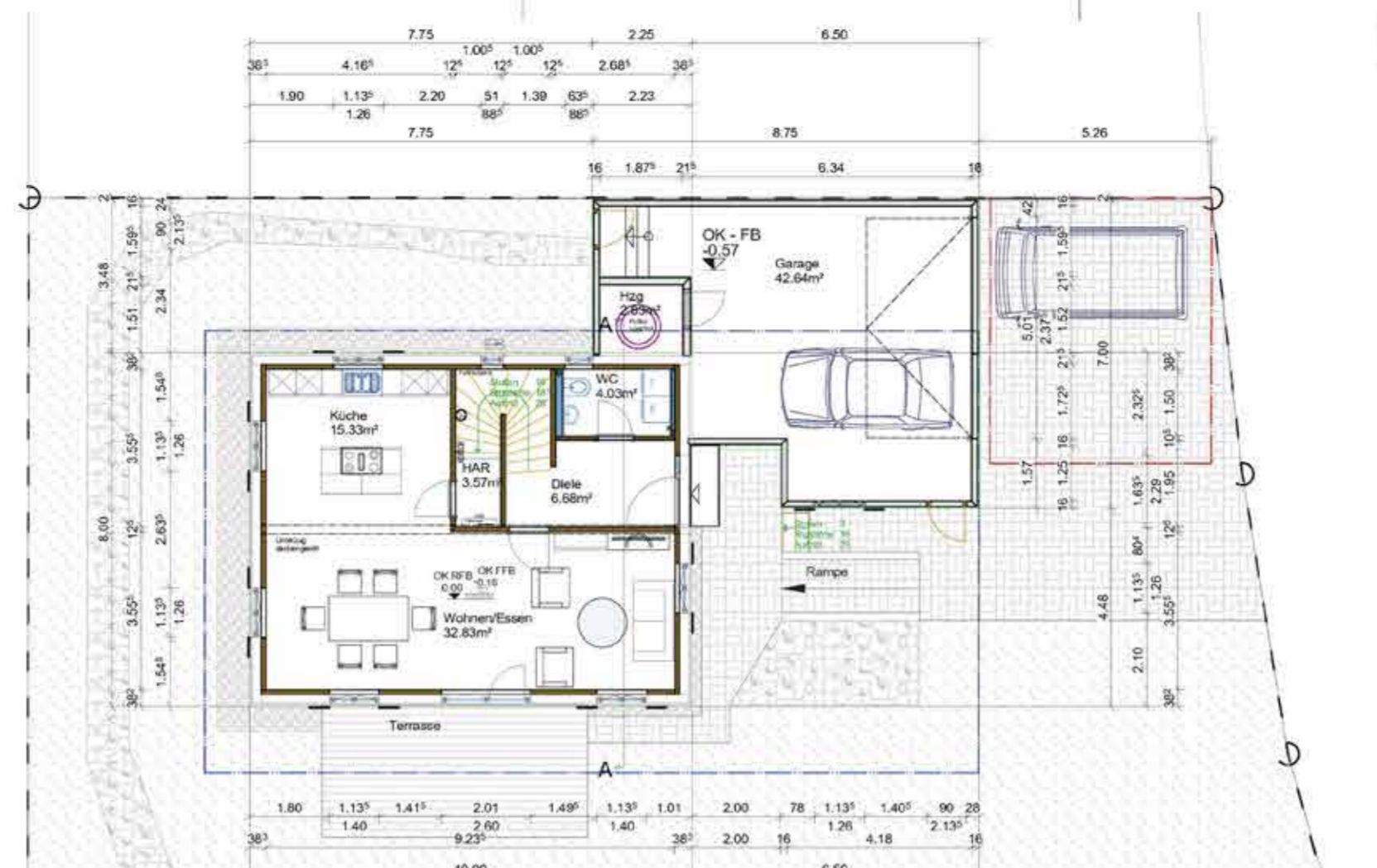
Erdgeschoss
