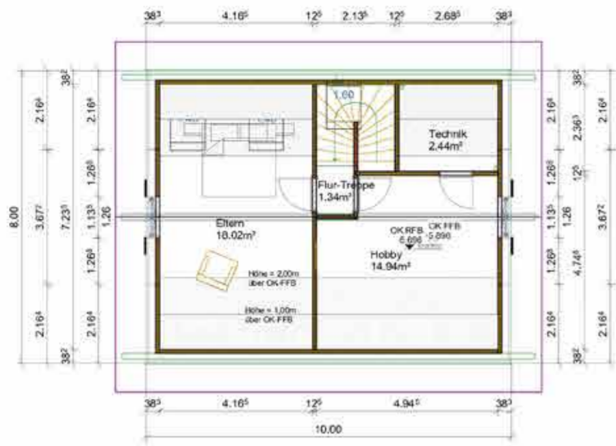
Dachgeschoss
