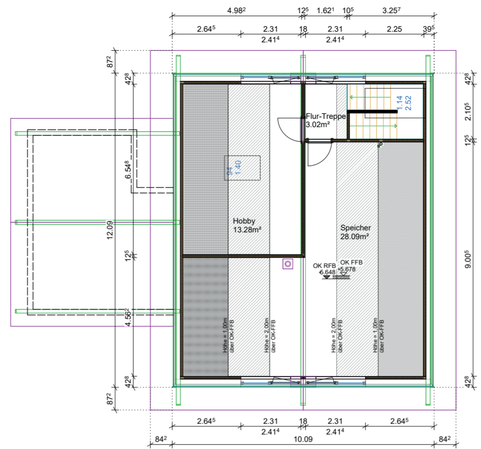
Dachgeschoss
