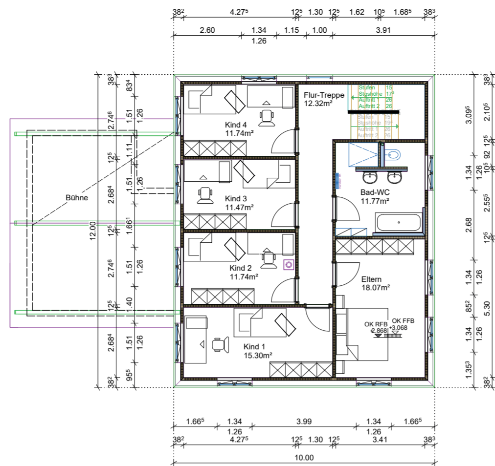
Obergeschoss
